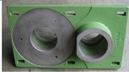
H.0310.01.1 Lagerplatte
